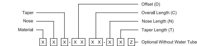
OFFSET NOSE (D)
